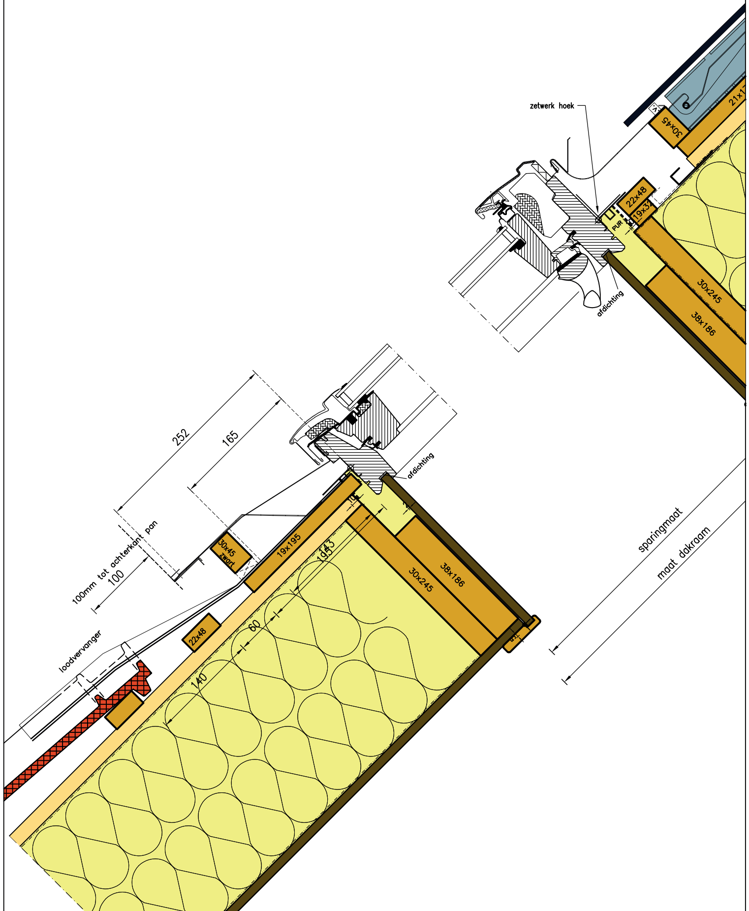
N7b dakraam onderaansluiting pannen
