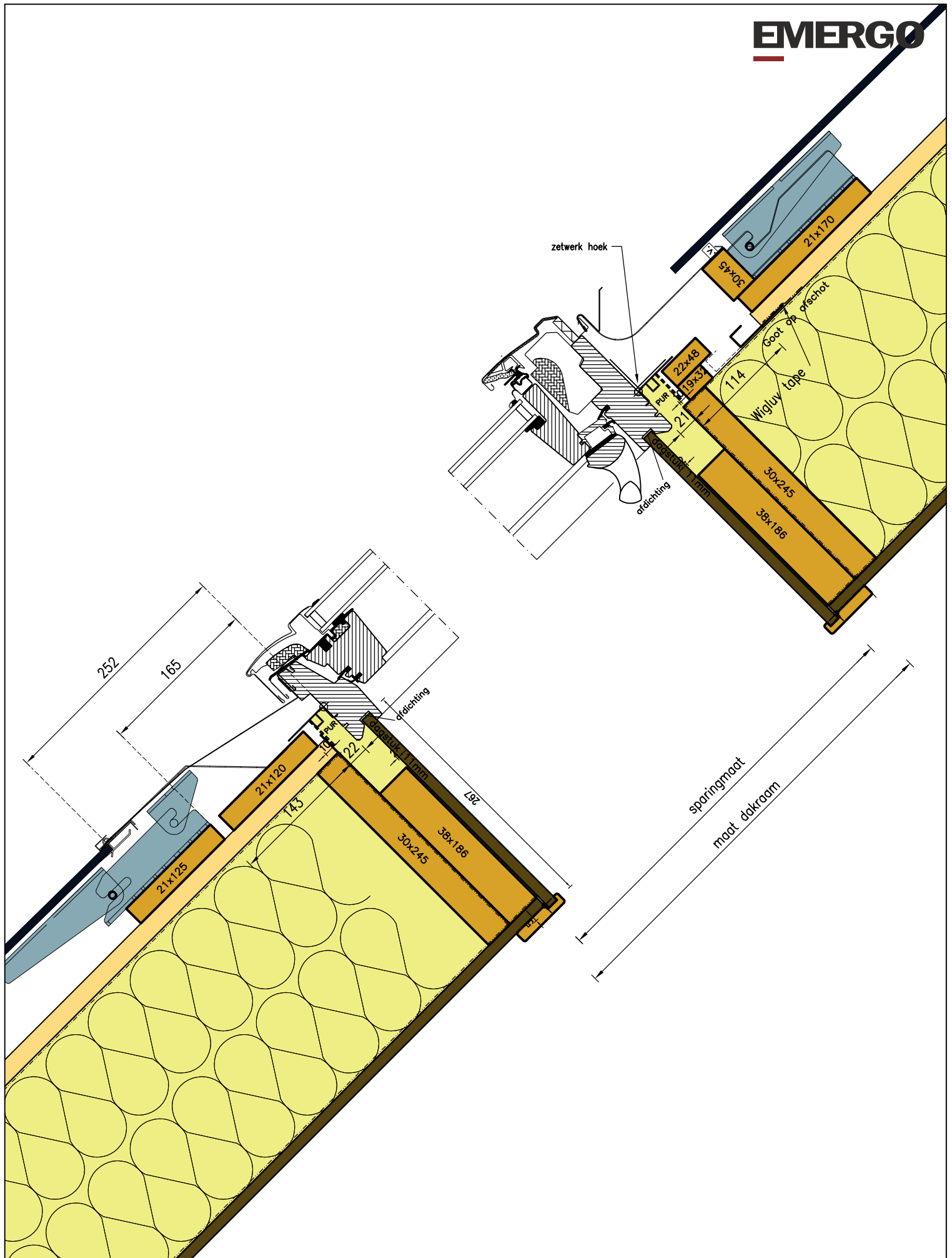
N7a dakraam boven- en onderaansluiting Navitect II
