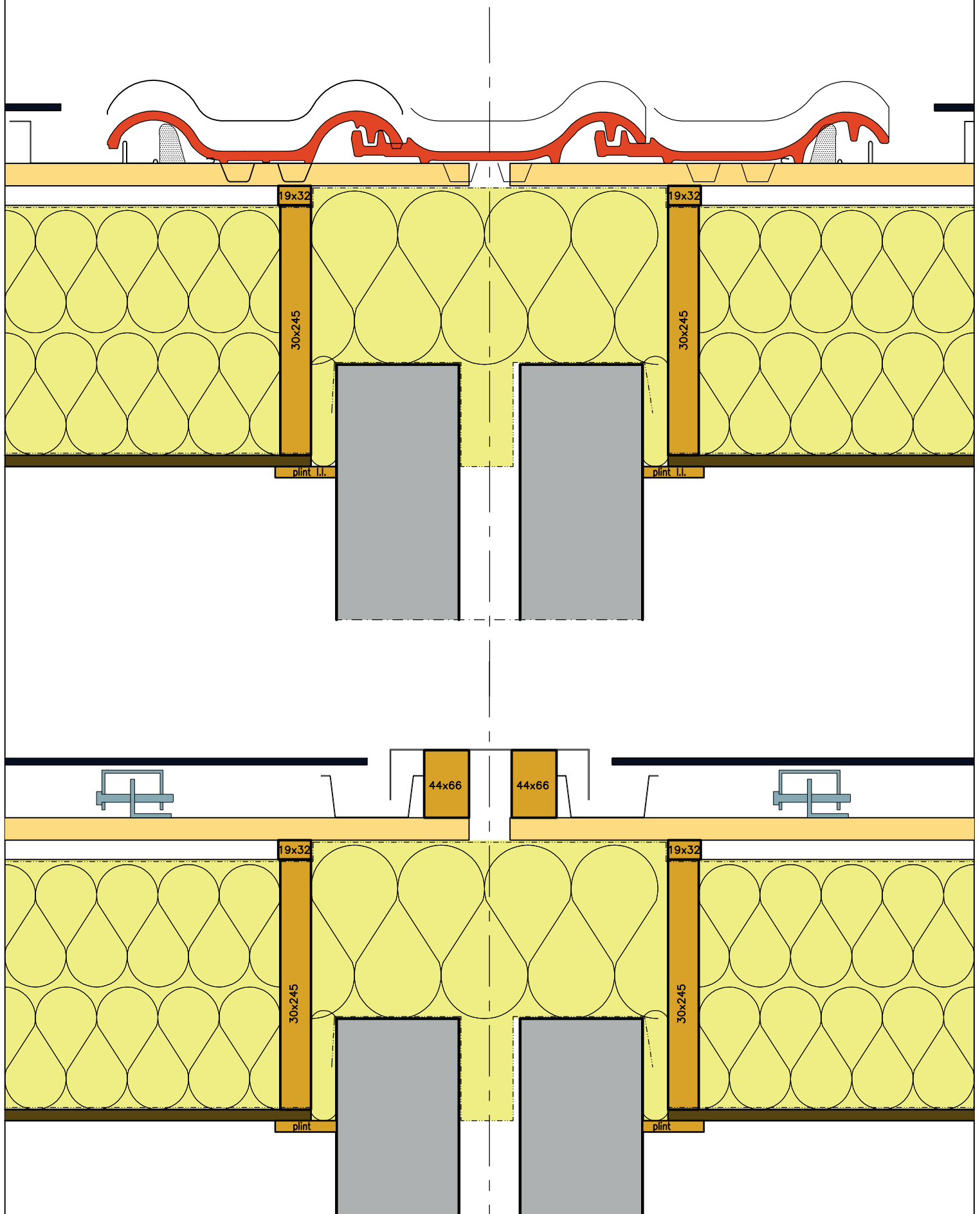
N6 oplossingen woningscheidende wand
